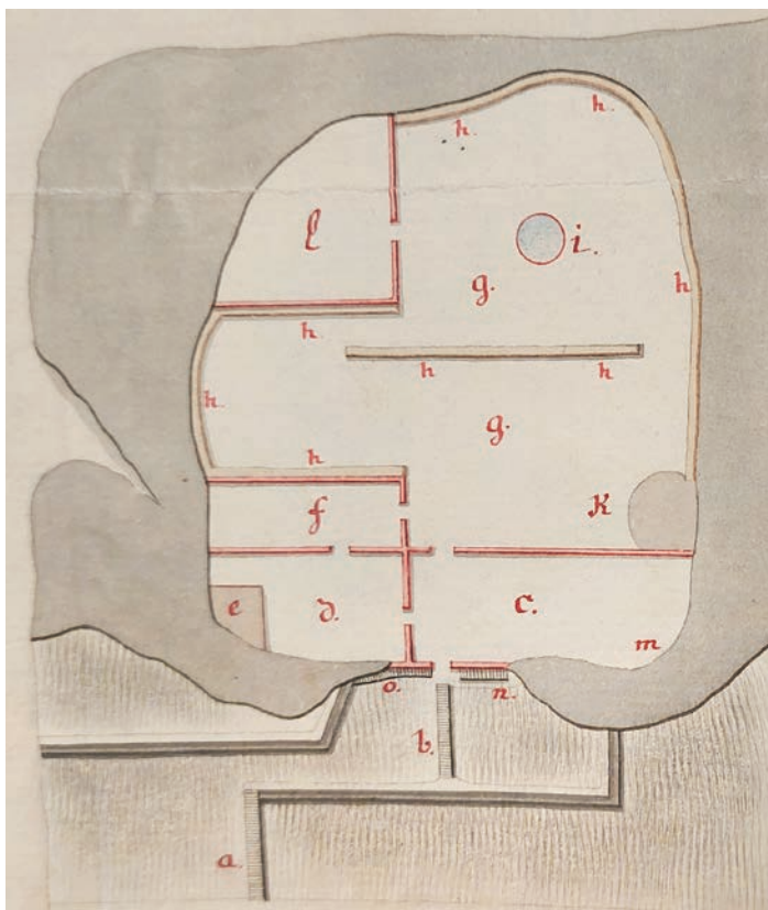
2. kép: A Veteráni-barlang és védműveinek alaprajza. C) pince, G) barakk, L) lőporraktár, K) sütőkemence (ÖSTA KA AFA 1788-13-ad1)
